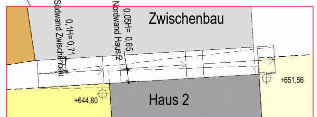
Ausschnitt Lageplan M 1 : 200
